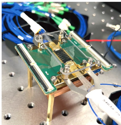
氮化硅集成光量子芯片。
